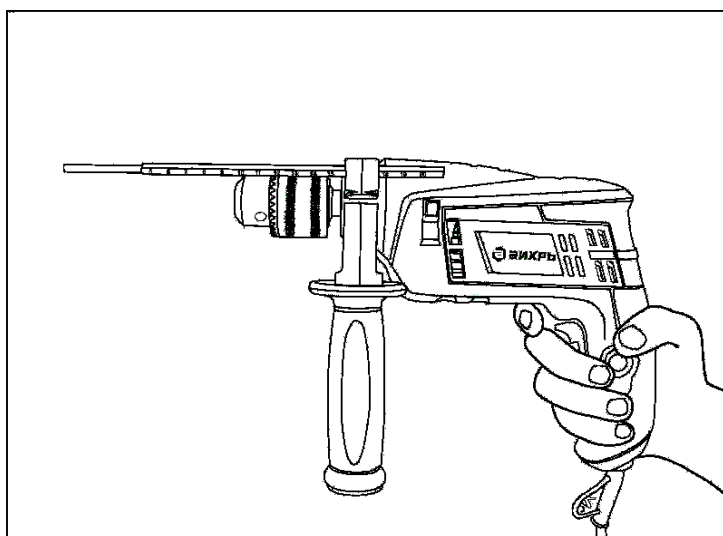
Рис. 5. Установка ограничителя сверления
