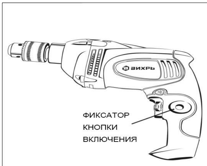
Рис. 8. Фиксатор кнопки включения
